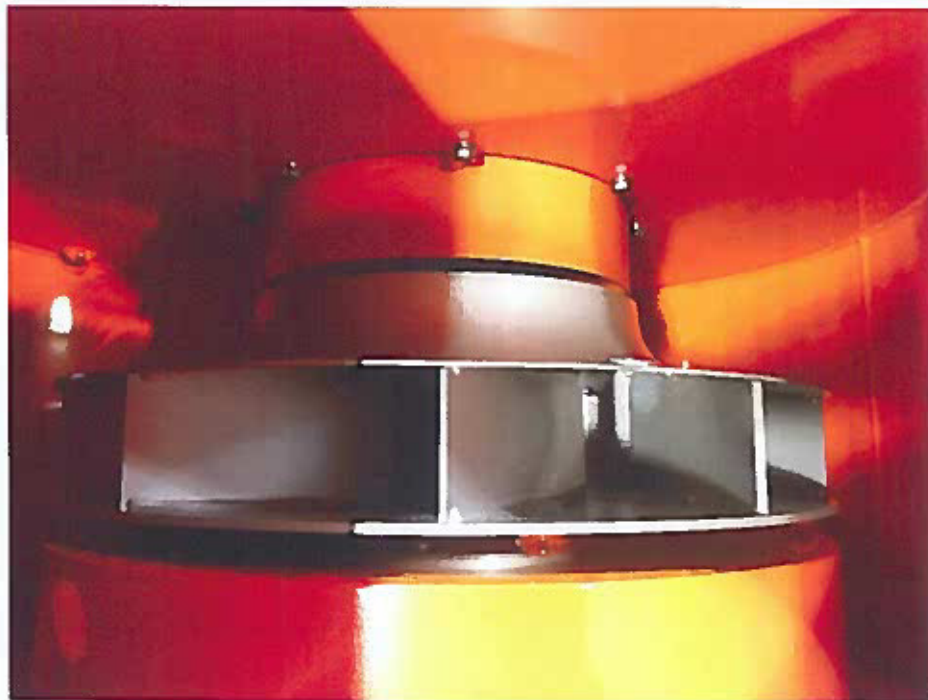
Фото 5 – Вид на рабочее колесо
