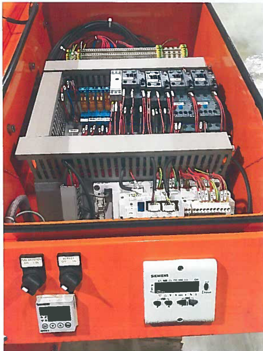
Фото 8- Общий вид на шкаф управления горелочным устройством
